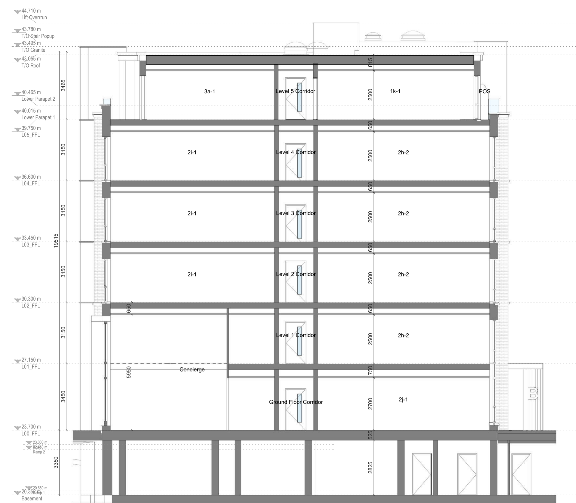
1 Section 1 1 : 100
