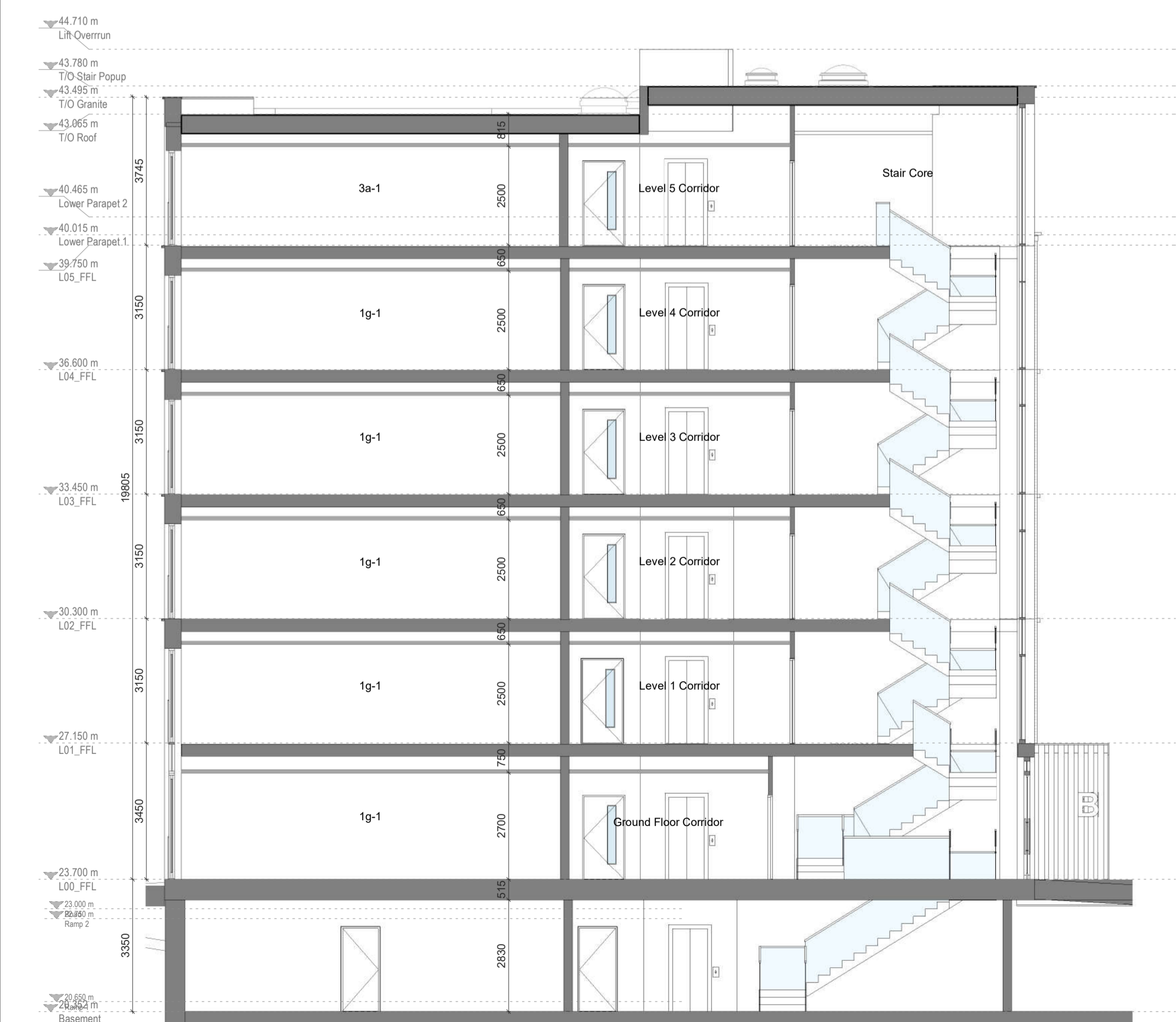
2 Section 2 1 : 100
