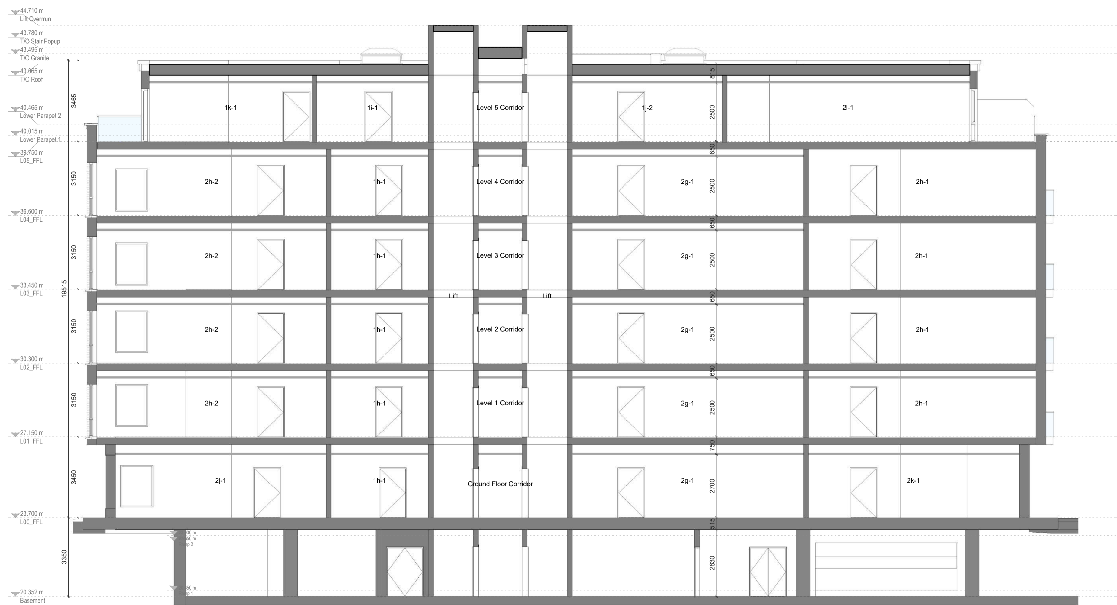
3 Section 3 1 : 100
